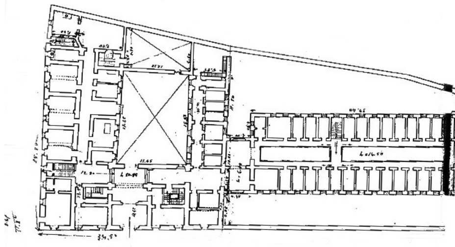
Fabbricato sede del Carcere Giudiziario di Oristano Pianta del piano terreno Scala 1:200
