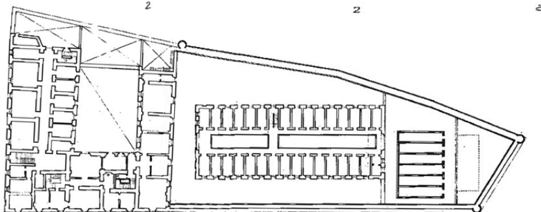
Fabbricato sede del Carcere Giudiziario di Oristano Pianta del primo piano Scala 1:200
