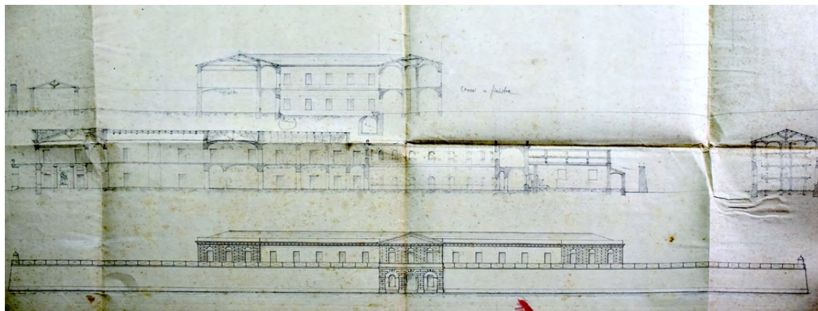
Figure 10a-b. Progetto di ampliamento del carcere "La Rotonda". di Timpio Pausania, dicembre 1862. A sinistra, (a) Pian Terreno; sotto, (b) Sezione Longitudinale e Prospetto principale. ASGCS, cart. 1/116, Carceri Giudiziarie di Timpio, 1/A, Disegni.
